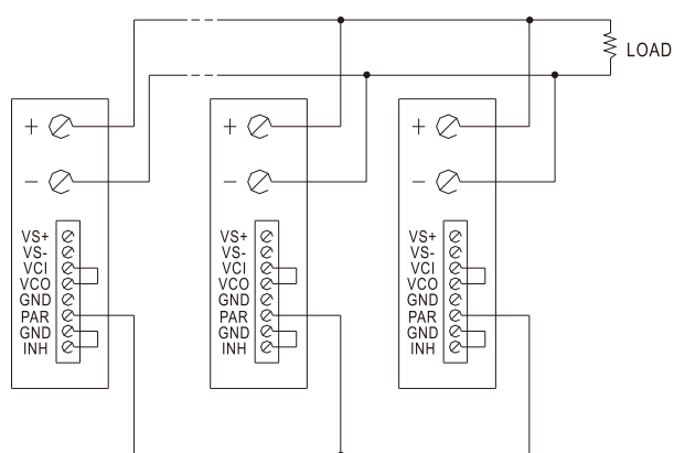
并联工作
