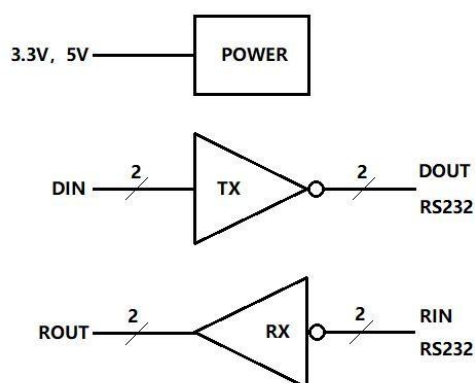
图2: SP3232A 逻辑图
