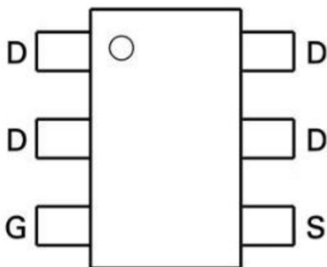
SOT23-6
