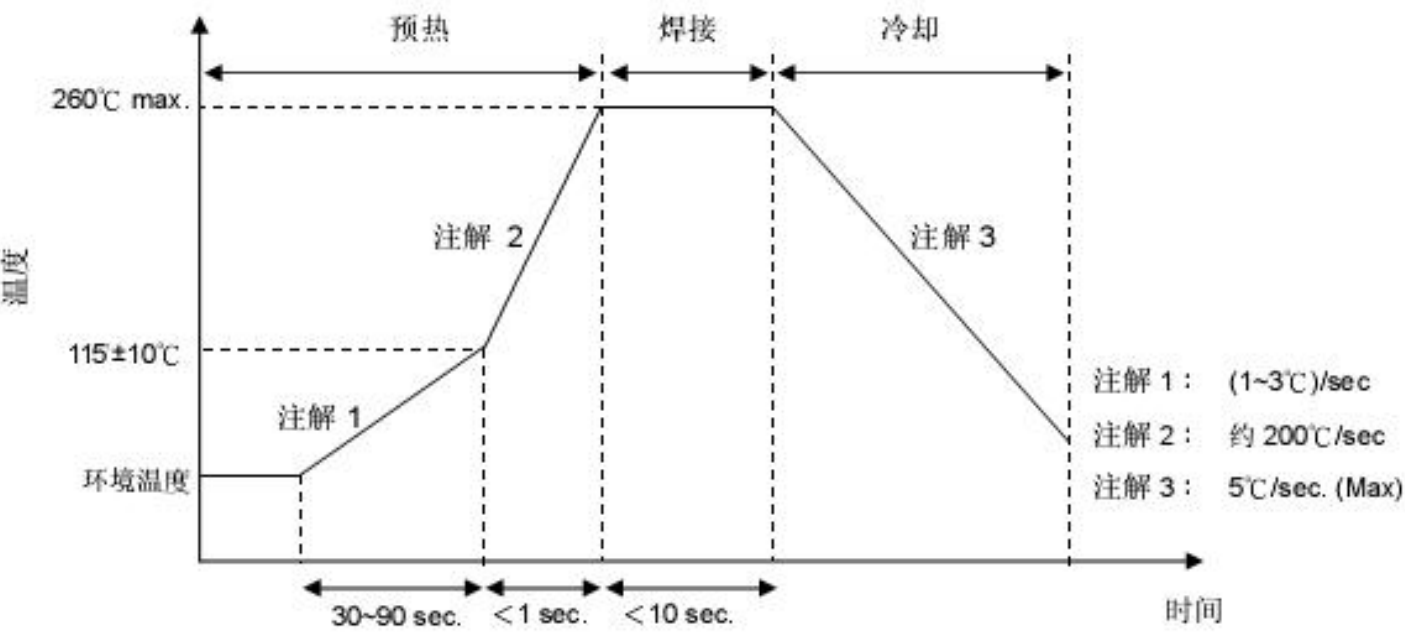
波峰焊曲线
