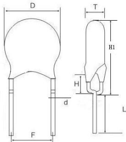
外形尺寸图
