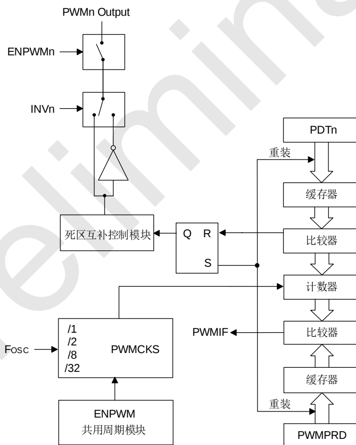
SC92F741X PWM 结构框图
