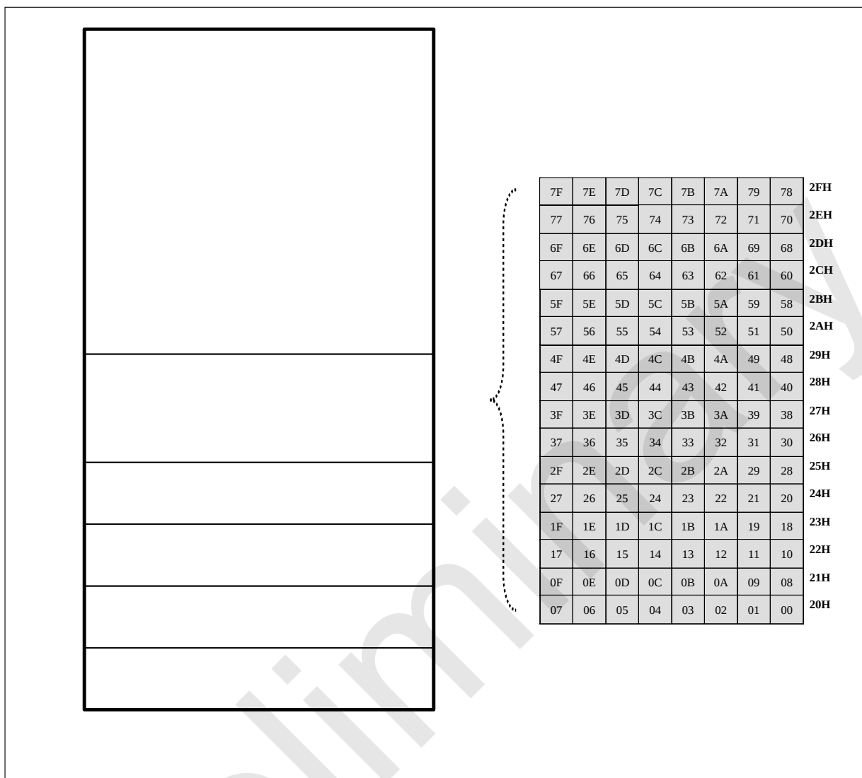
SRAM 结构图
