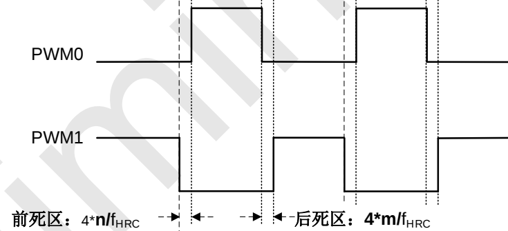
PWM 死区输出波形
