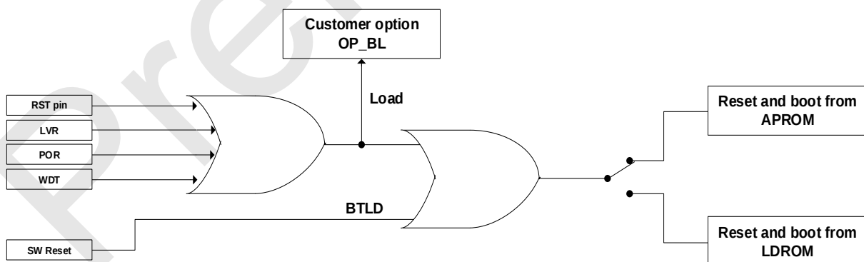
SC95F852X 复位后启动区域切换示意图
