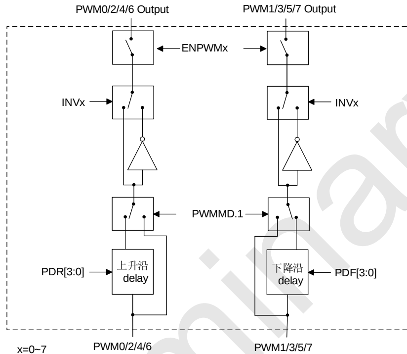
SC95F852X PWM 互补模式框图
