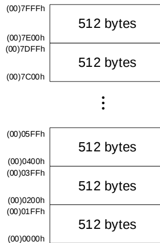
SC95F852X 32 Kbytes Flash ROM Sector 分区示意
