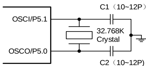
32.768kHz 外部晶振连接图
