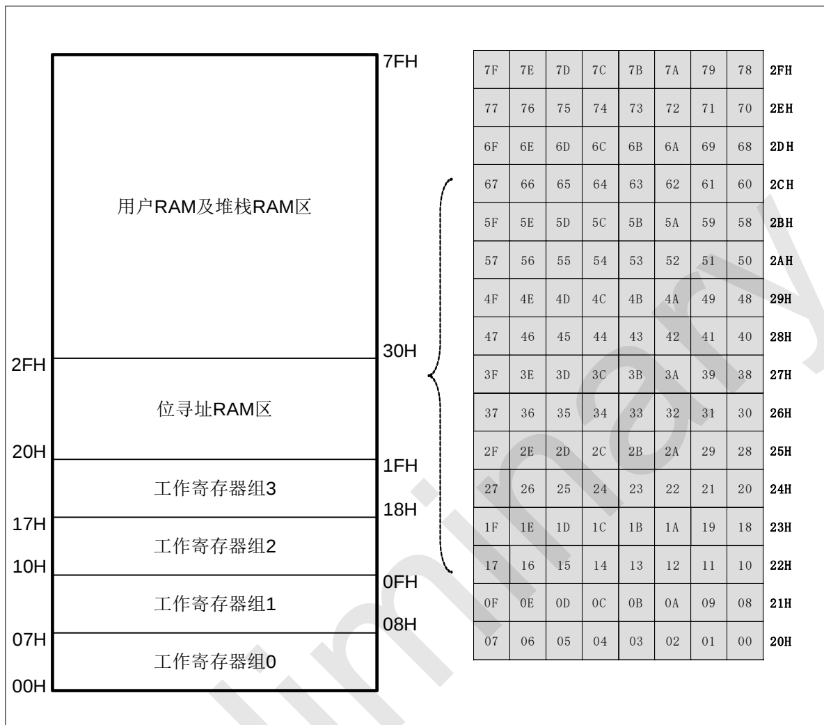
SRAM 结构图
