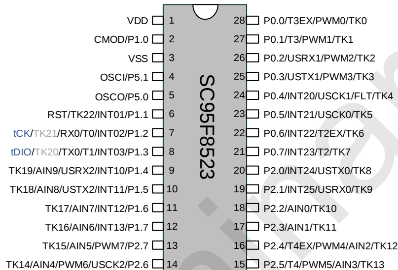
SC95F8523 管脚配置图
