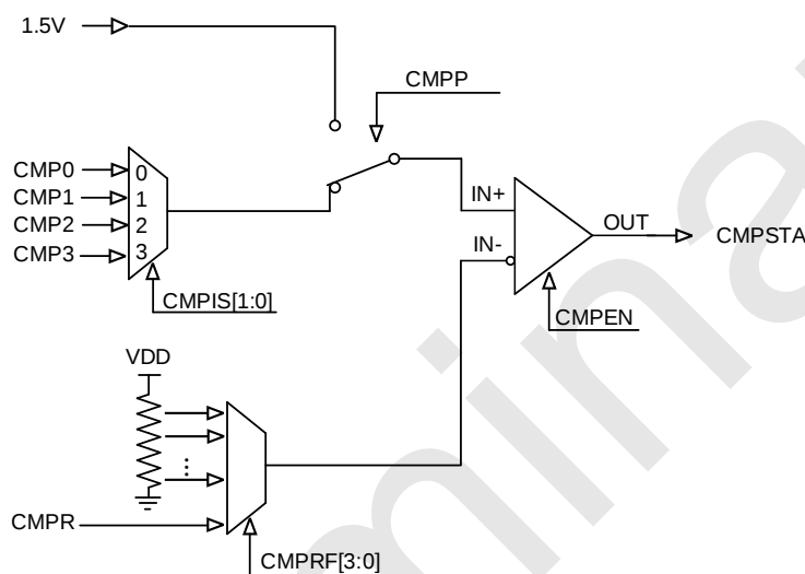
模拟比较器结构框图
