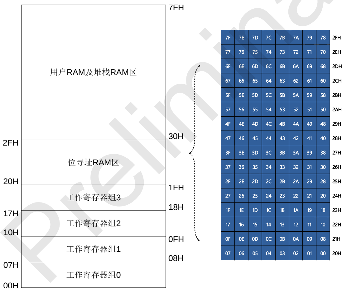
SRAM 结构图
