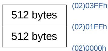
SC92F759X EEPROM Sector 分区示意
