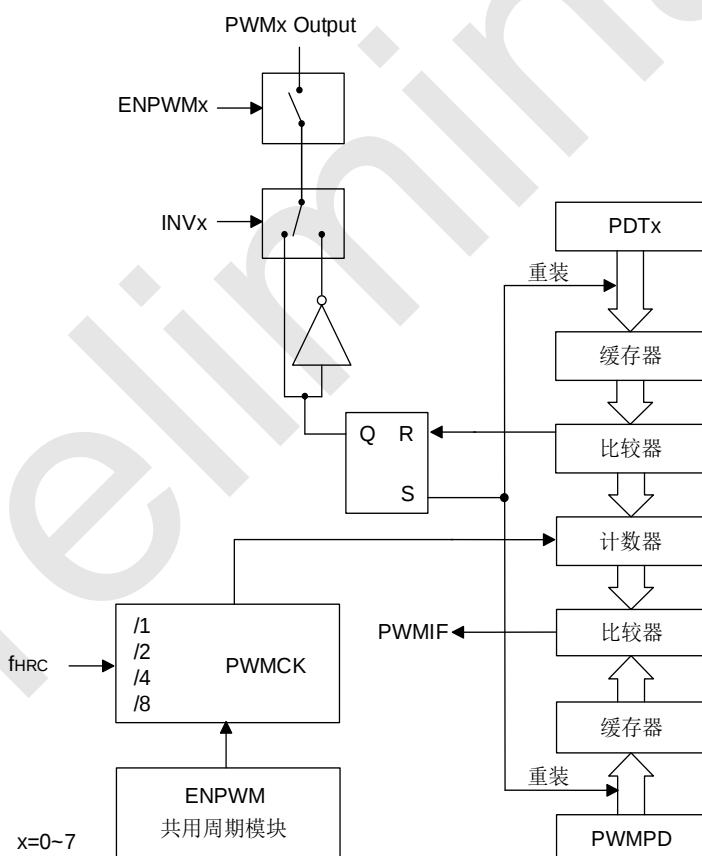
SC92F759X PWM 结构框图
