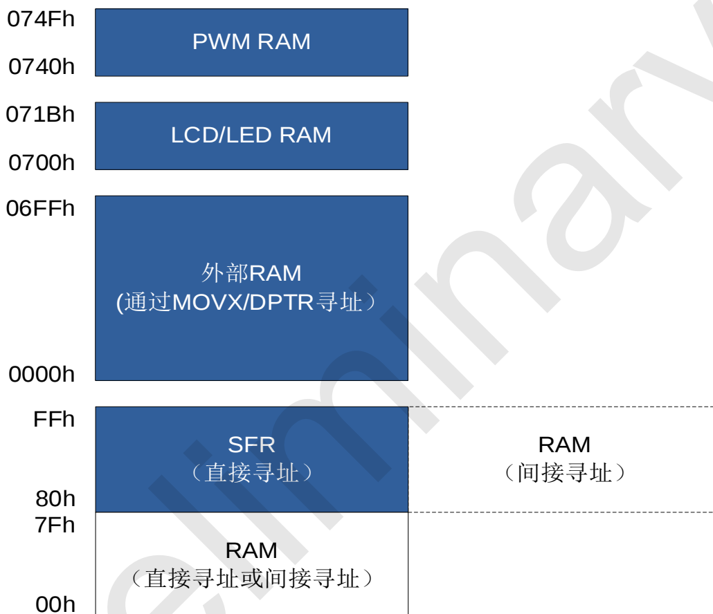
SRAM 结构图
