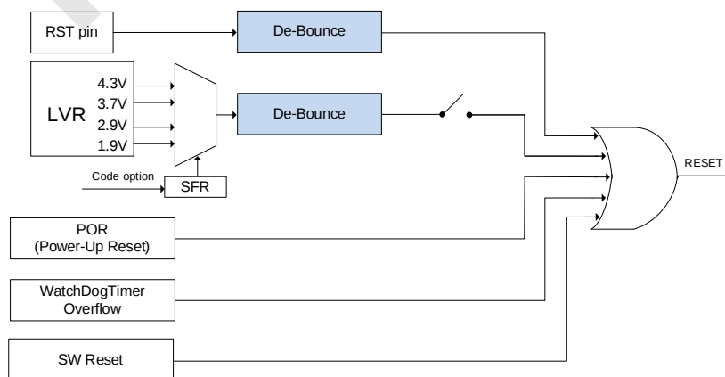
SC92F759X 复位电路图
