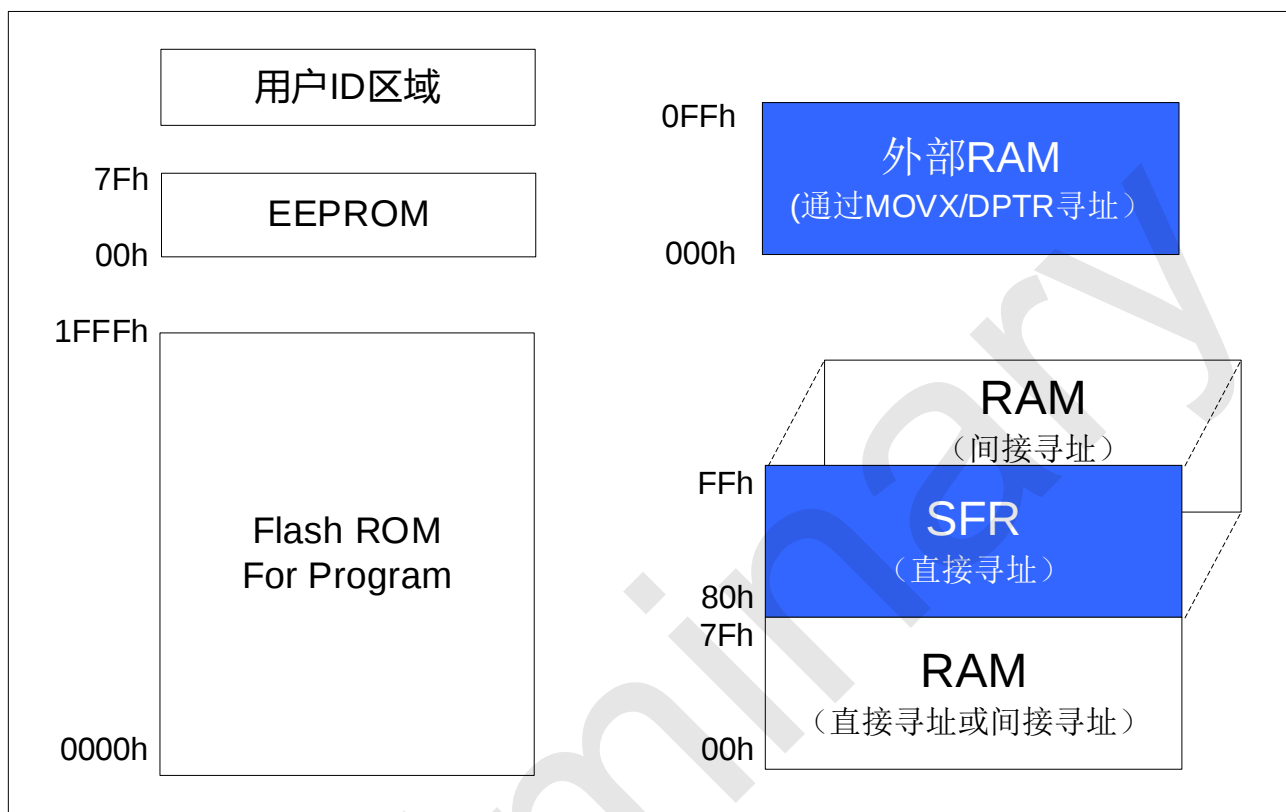
Flash ROM 和 SRAM 结构图
