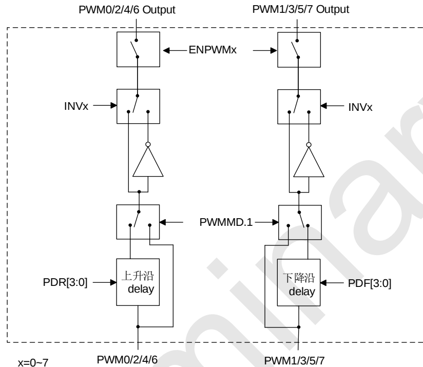
SC92L853X PWM 互补模式框图
