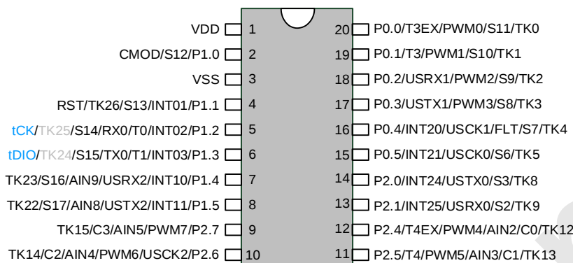
SC92L8532 管脚配置图（SOP20/TSSOP20）
