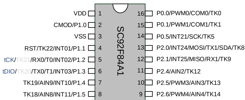
SC92F84A1 管脚配置图
