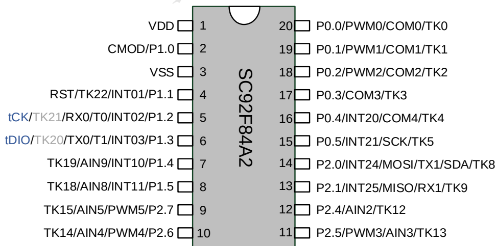
SC92F84A2 管脚配置图
