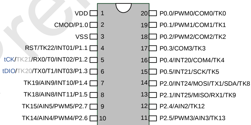
SC92F8412 管脚配置图 适用于 SOP20/TSSOP20 封装
