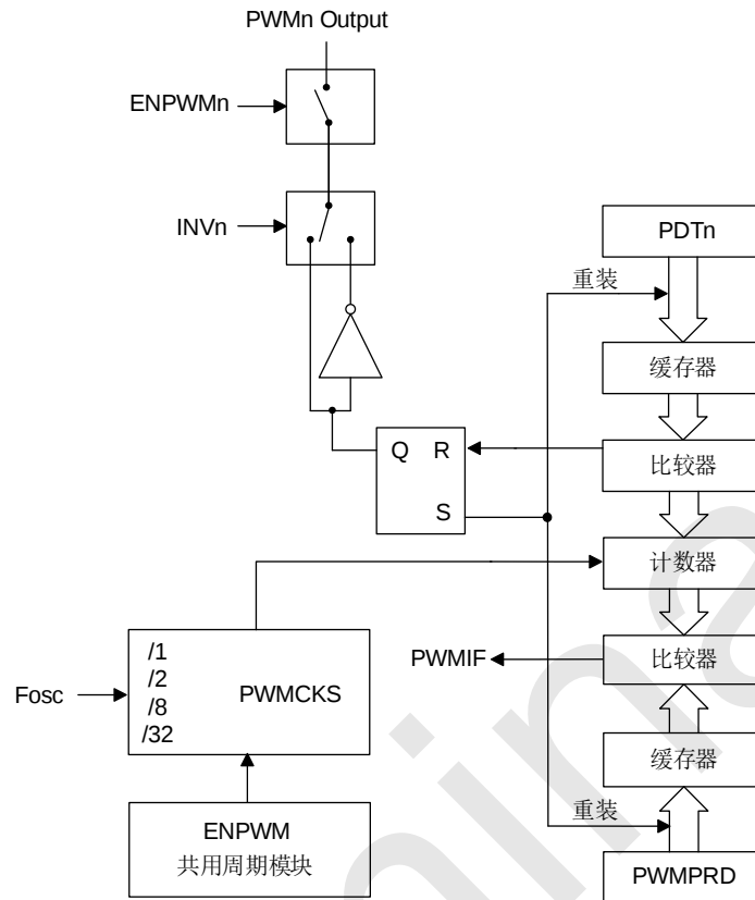
SC92F841X PWM 独立模式框图
