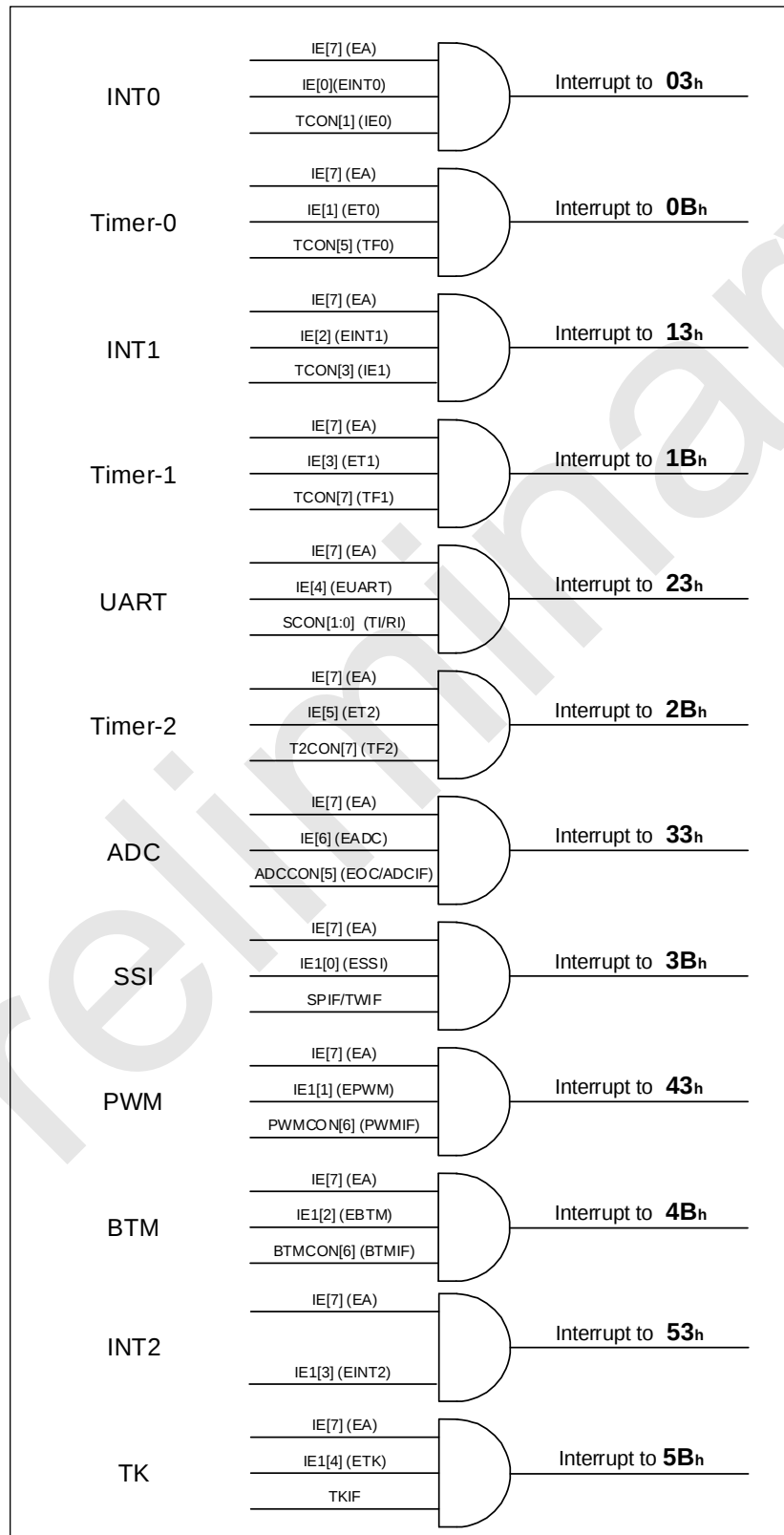
SC92F841X 中断结构和向量
