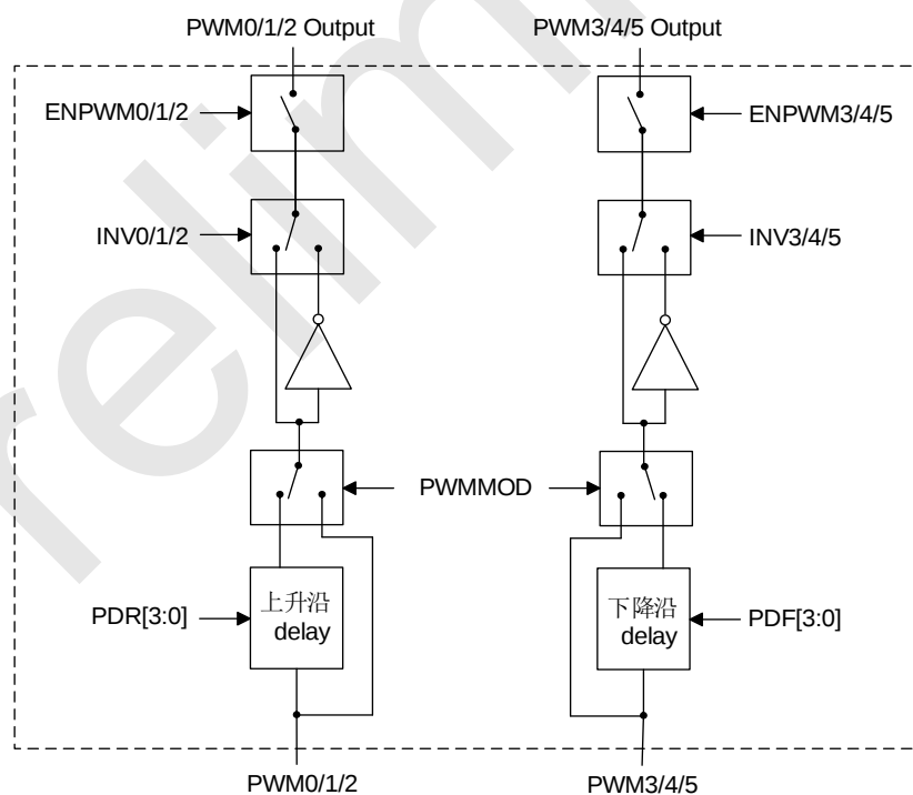
SC92F841X PWM 互补模式框图
