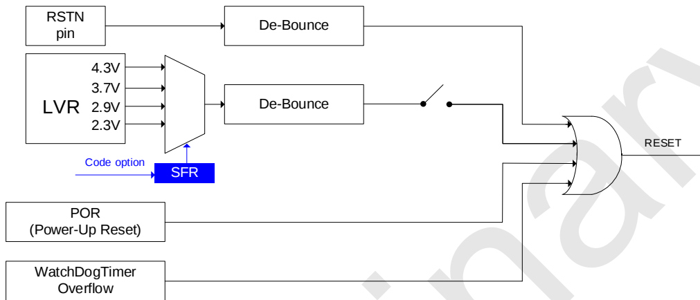
SC92F841X 复位电路图
