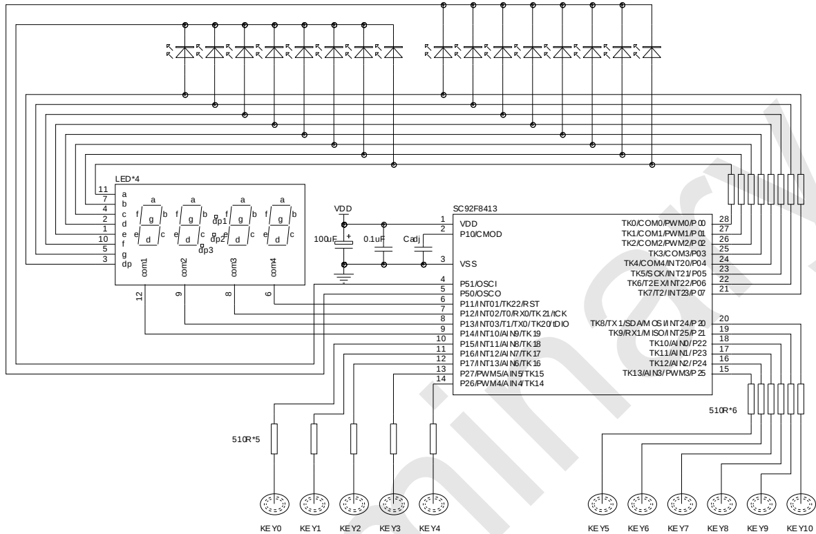
SC92F8413 Touch Key 应用电路图
