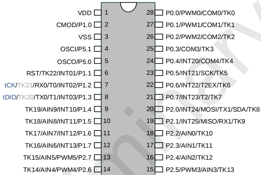
SC92F8413 管脚配置图 适用于 SOP28/TSSOP28 封装
