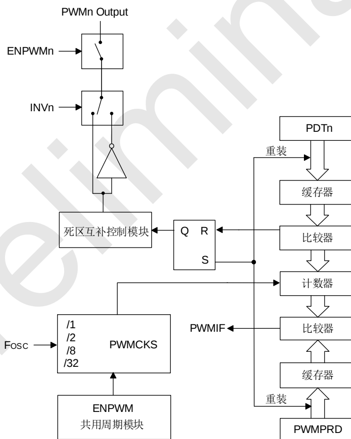
SC92F841X PWM 结构框图
