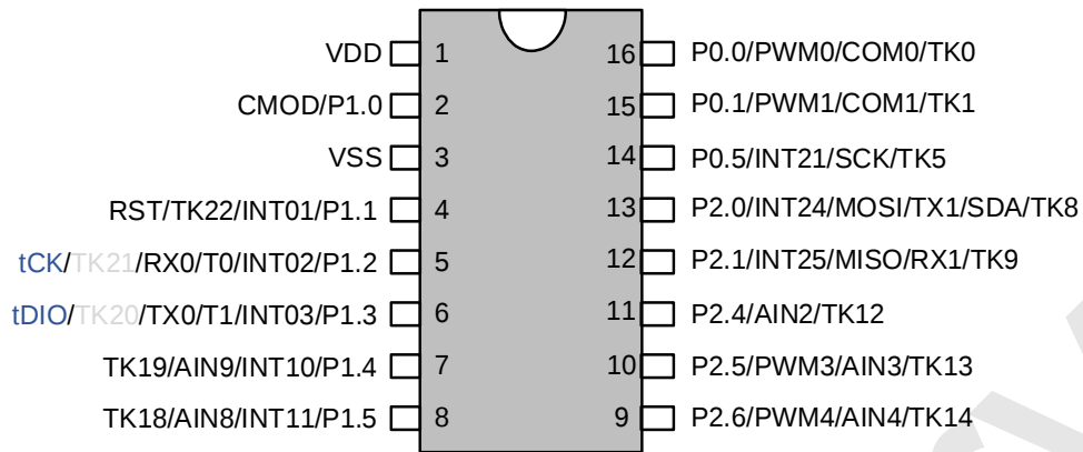
SC92F8411 管脚配置图 适用于 SOP16 封装
