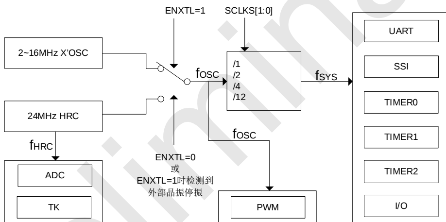
SC92F841X 内部时钟关系
