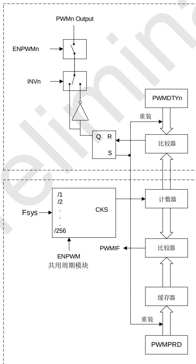
SC92F720X PWM 结构框图
