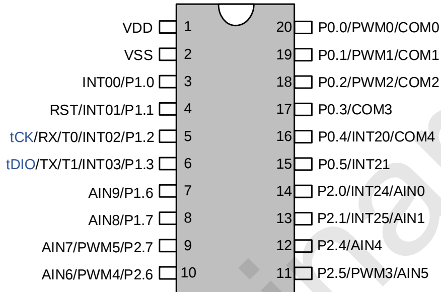
SC92F7202 管脚配置图 适用于 SOP20/TSSOP20 封装
