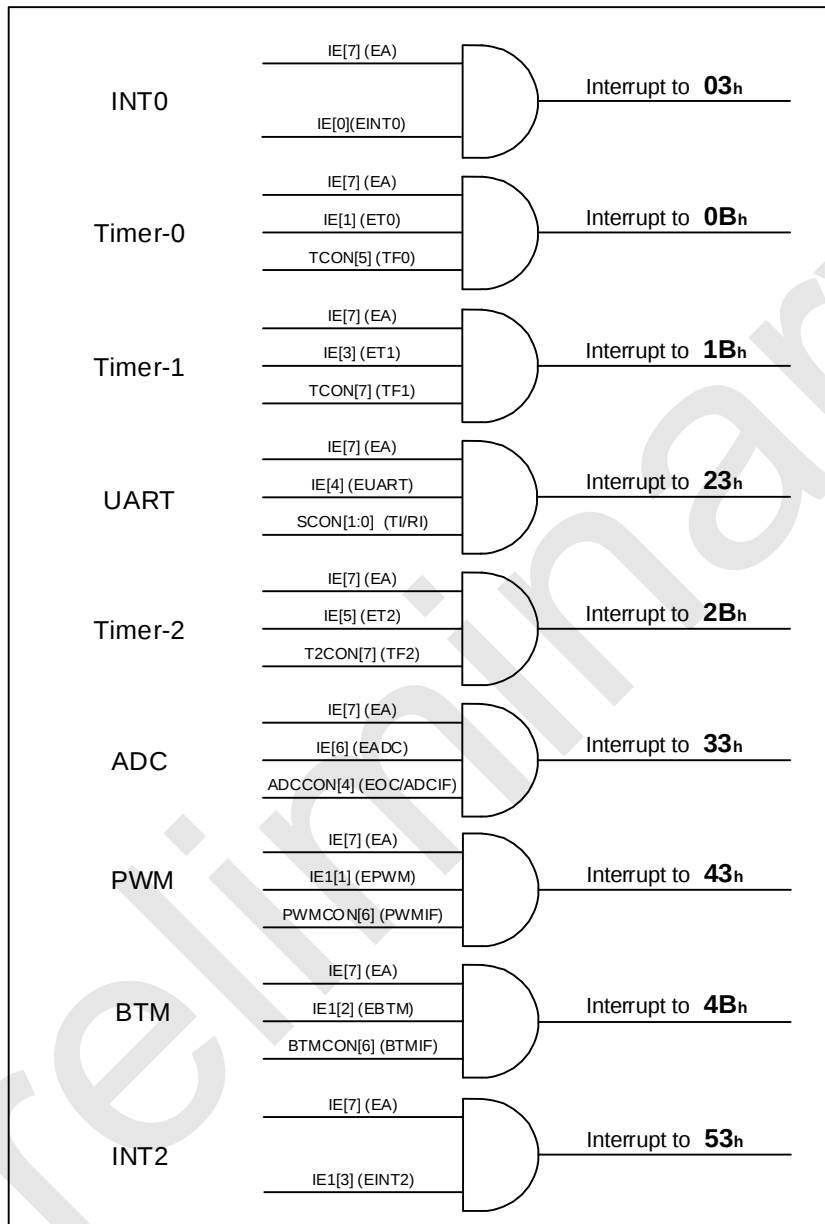
SC92F720X 中断结构和向量
