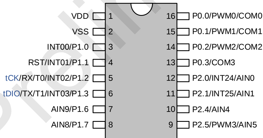
SC92F7201 管脚配置图 适用于 SOP16 封装
