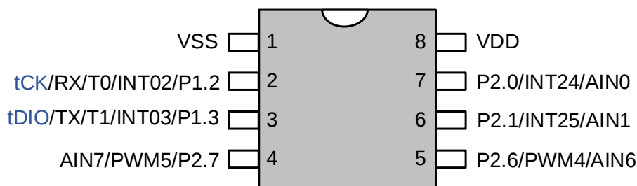
SC92F7200 管脚配置图 适用于 SOP8 封装
