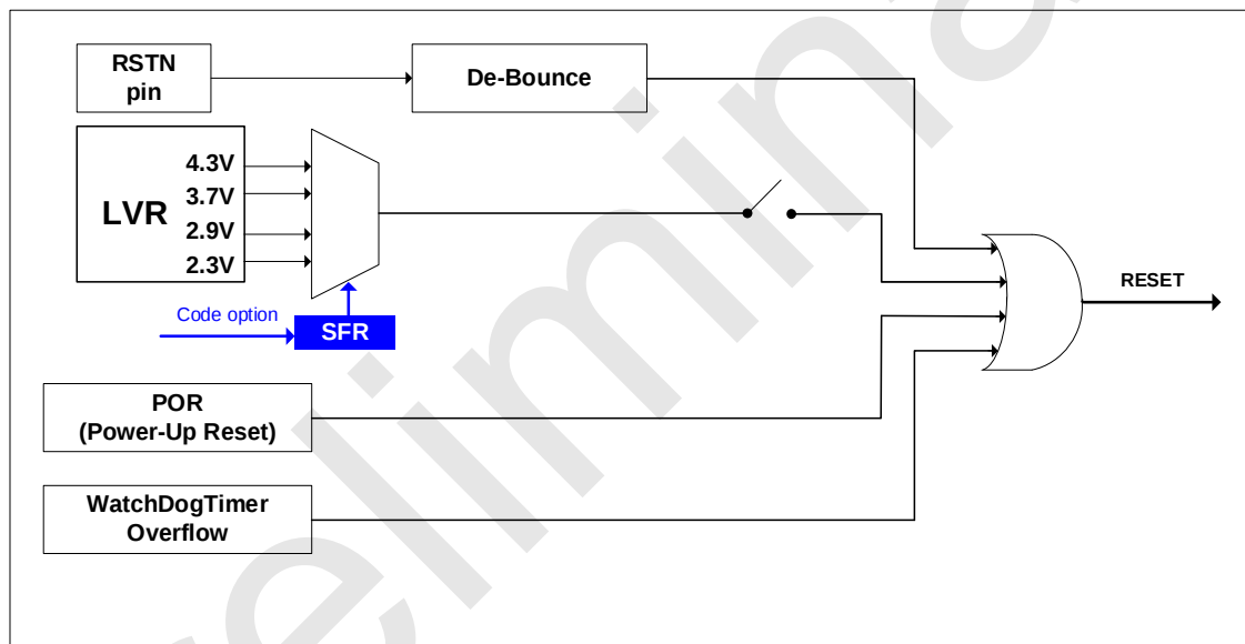
SC92F720X 复位电路图
