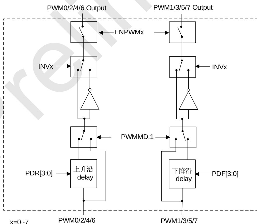
SC95F861XB PWM 互补模式框图
