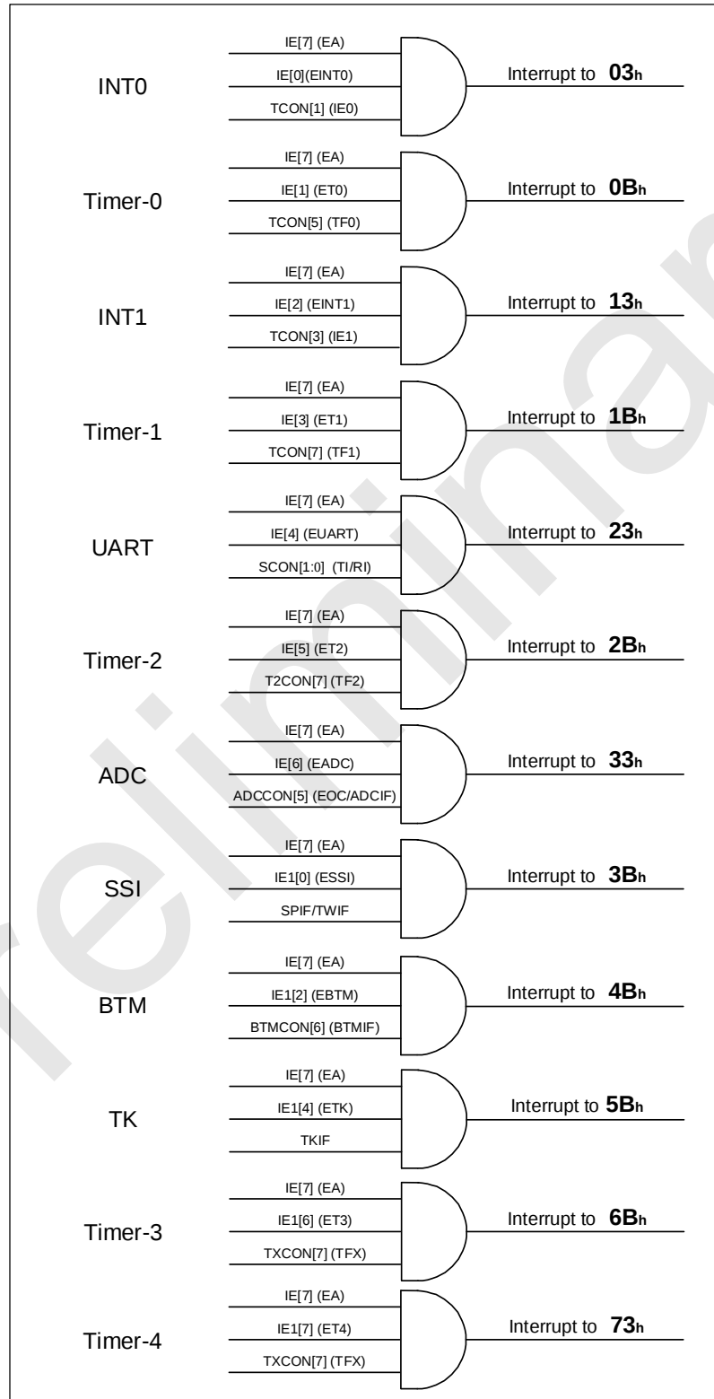
SC92F84HX 中断结构和向量
