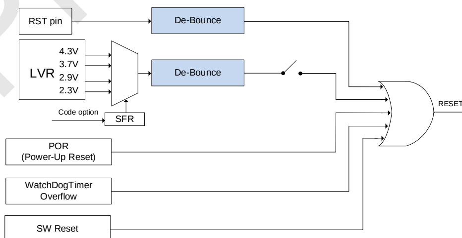
SC92F84HX 复位电路图
