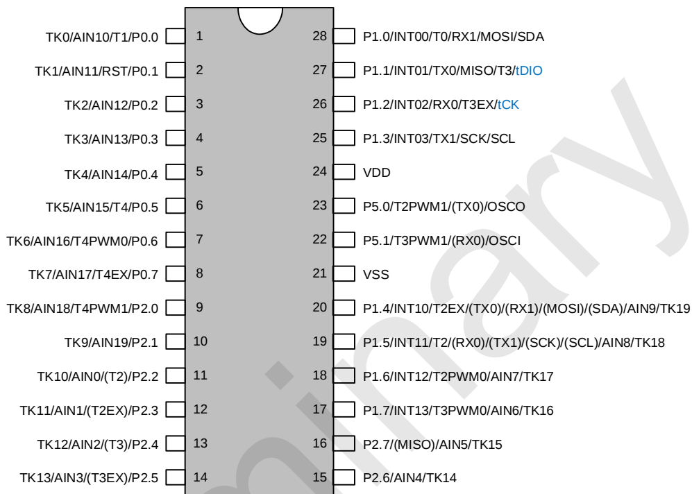
28PIN 管脚配置图 适用于 SOP28、TSSOP28 封装
