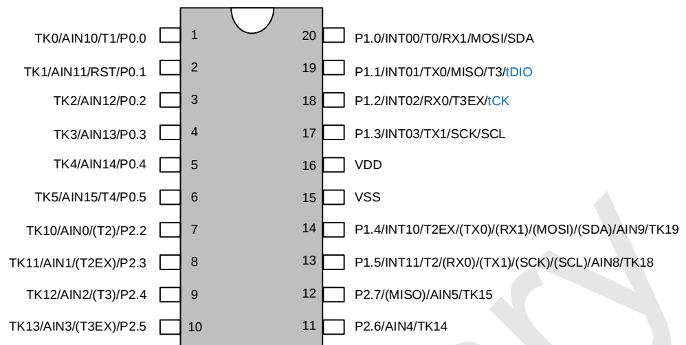
20PIN 管脚配置图 适用于 SOP20、TSSOP20 封装
