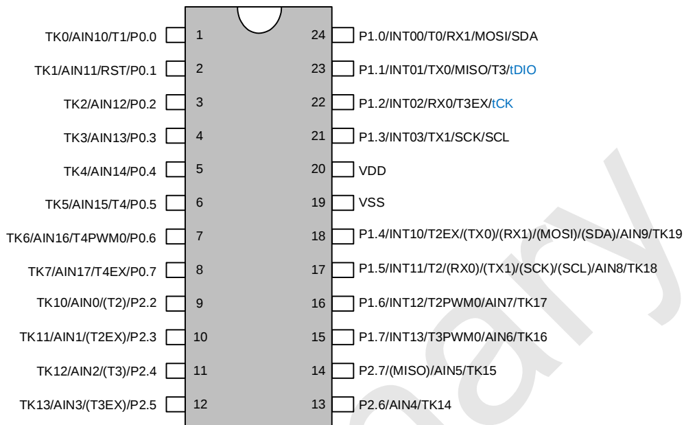
24PIN 管脚配置图 适用于 SOP24、TSSOP24 封装
