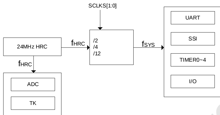
SC92F84HX 内部时钟关系
