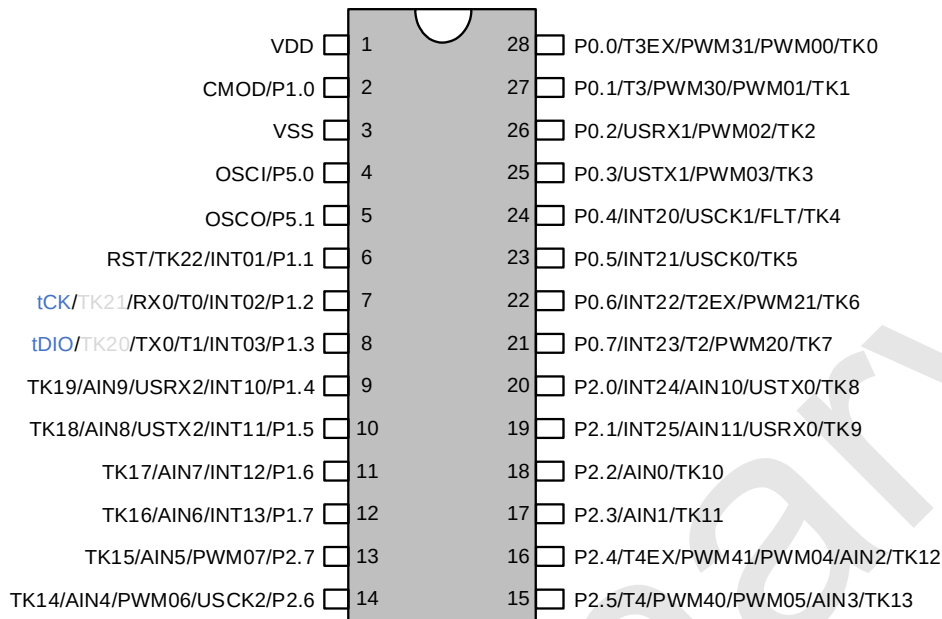
SC95F8573 管脚配置图 适用于 SOP28、TSSOP28 封装
