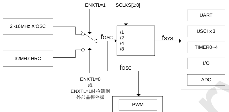
SC95F757X 内部时钟关系
