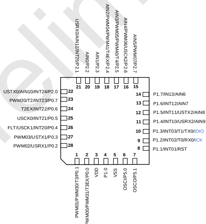
SC95F7573 管脚配置图 适用于 QFN28 封装
