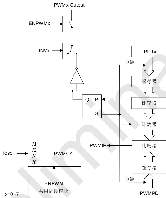
SC95F757X PWM 独立模式框图
