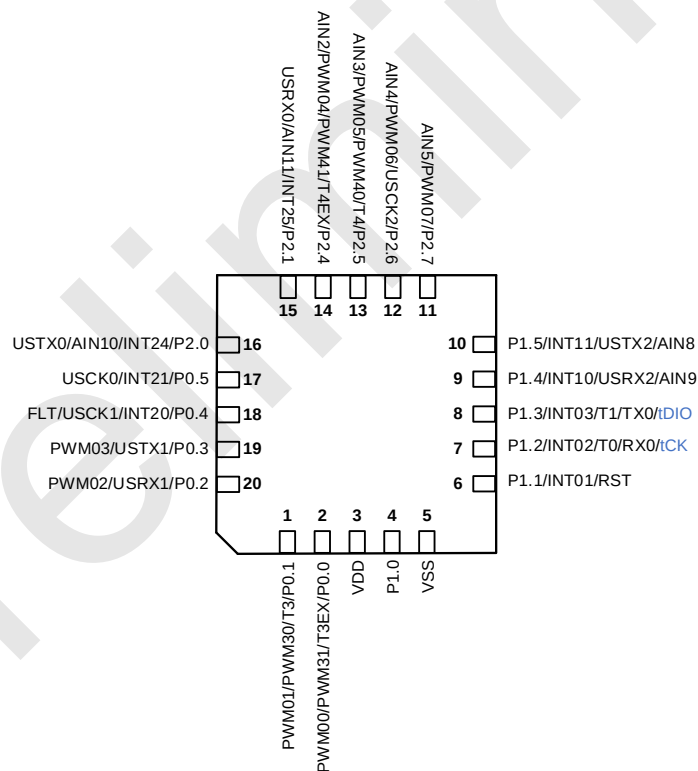
SC95F7572 管脚配置图 适用于 QFN20 封装
