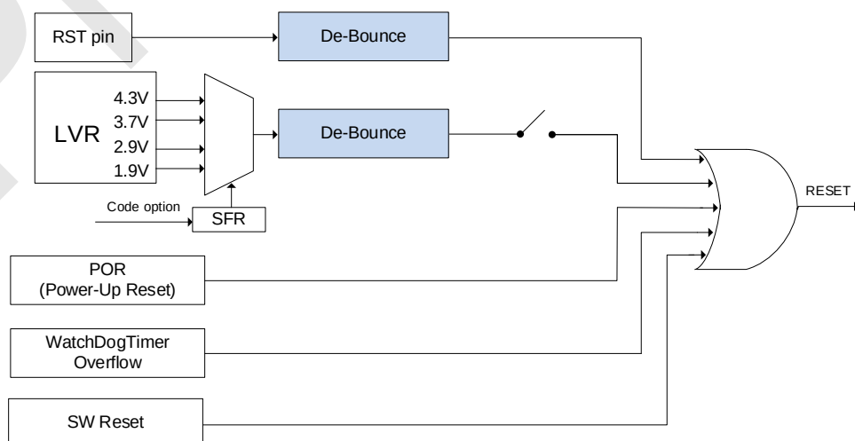
SC95F757X 复位电路图
