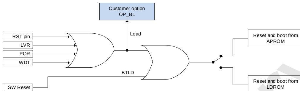
SC95F757X 复位后启动区域切换示意图
