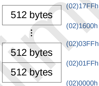
SC95F757X EEPROM Sector 分区示意
