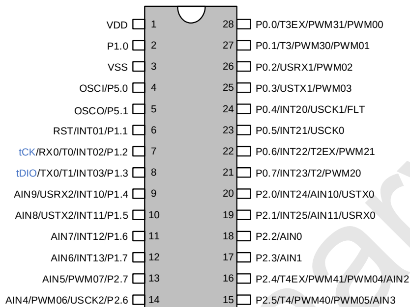
SC95F7573 管脚配置图 适用于 SOP28、TSSOP28 封装
