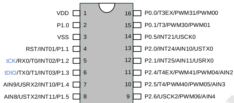
SC95F7571 管脚配置图 适用于 SOP16 封装
