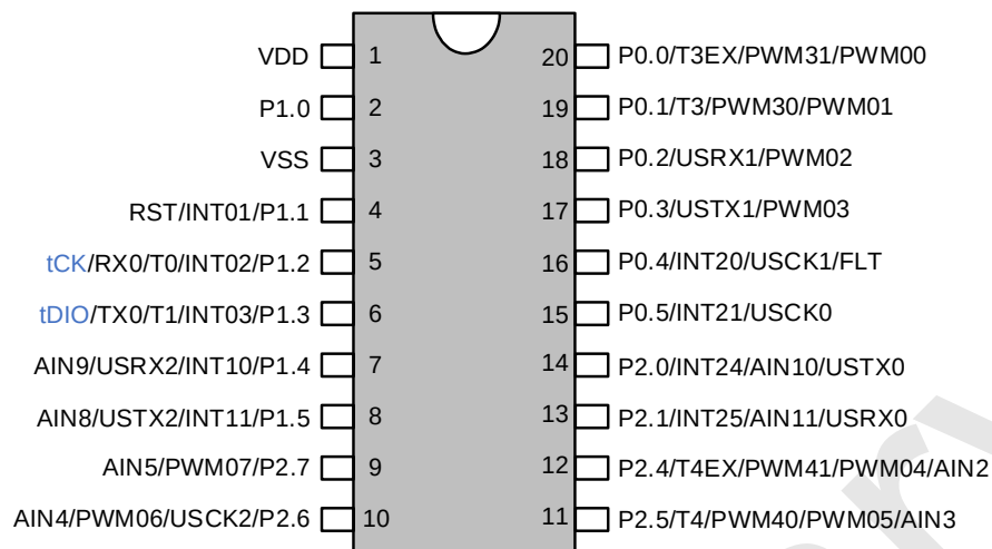
SC95F7572 管脚配置图 适用于 SOP20、TSSOP20 封装
