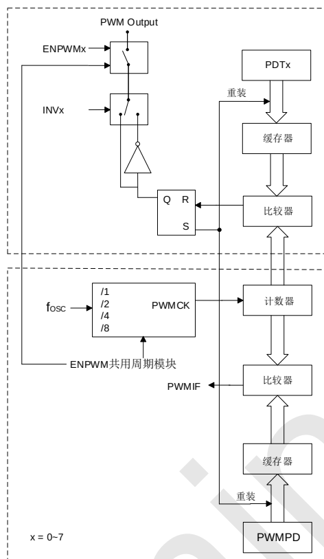
SC95F757X PWM 结构框图
