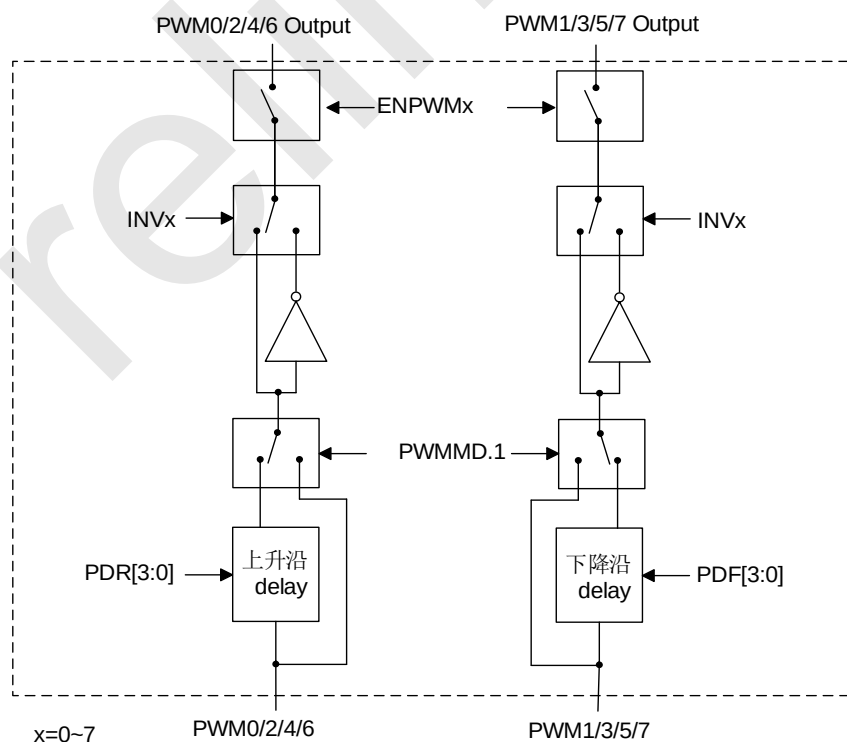
SC95F757X PWM 互补模式框图
