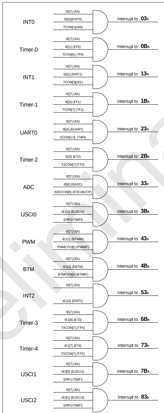
SC95F757X 中断结构和向量
