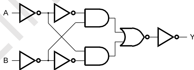
图 3 逻辑框图
