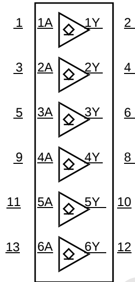
图 1 逻辑符号
