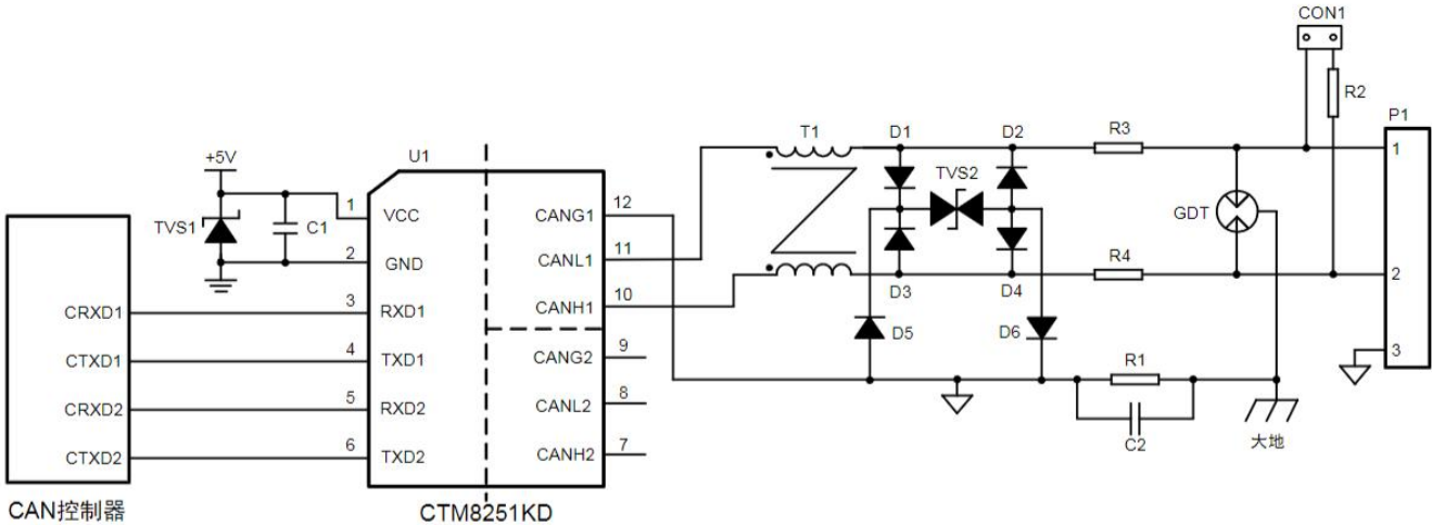
图 2. EMC 推荐电路
