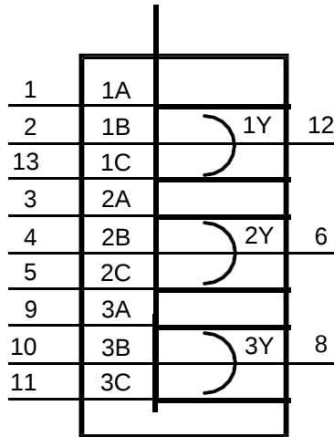
图 1 逻辑符号
