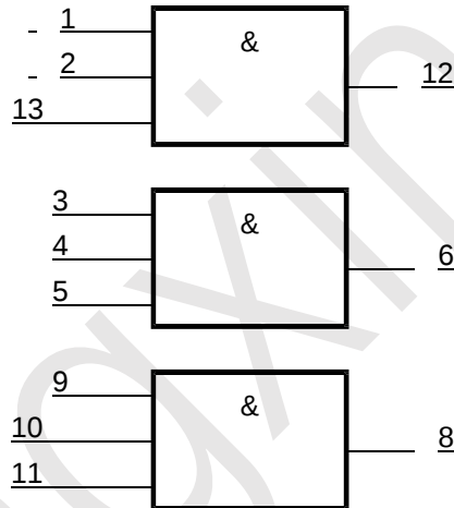
图 2 IEC 逻辑符号
