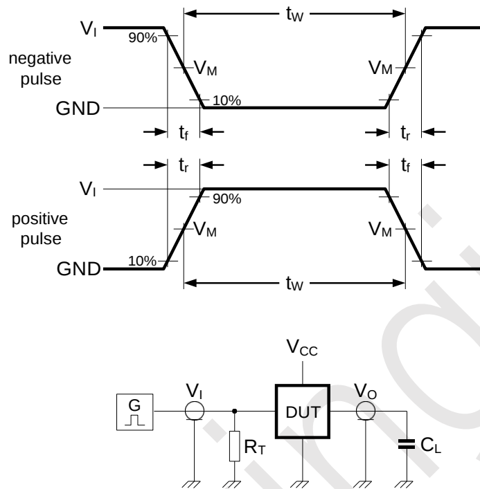
图4 测量开关时间的测试电路
