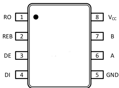
(b) MSOP8
