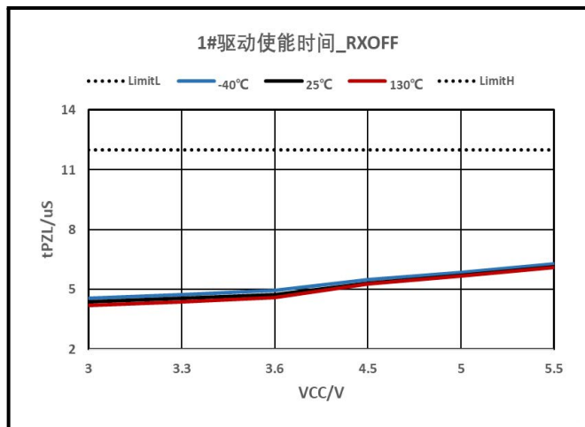
图 12: 驱动使能时间
