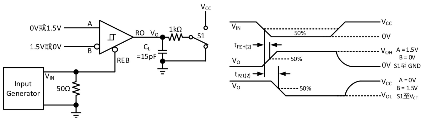
图 26: 在驱动器禁用情况下测量接收机使能时间
