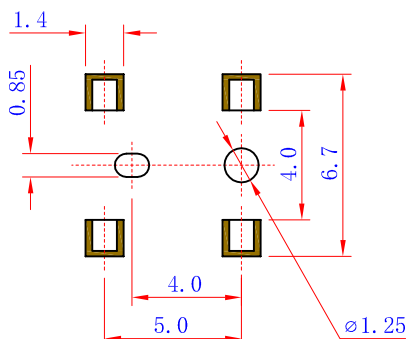
安装尺寸图
