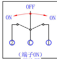
(端子ON) 回路图
