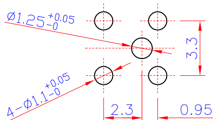
安装尺寸图
