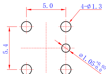
安装尺寸图
