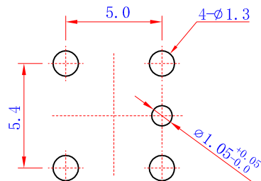
安装尺寸图
