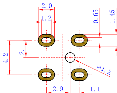
安装尺寸图
