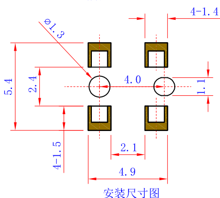
安装尺寸图
