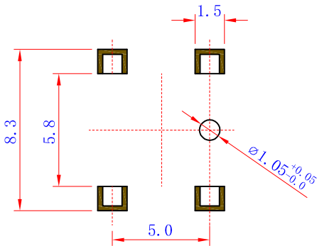
安装尺寸图
