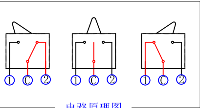
电路原理图
