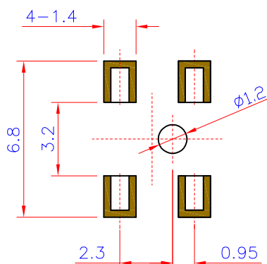
安装尺寸图
