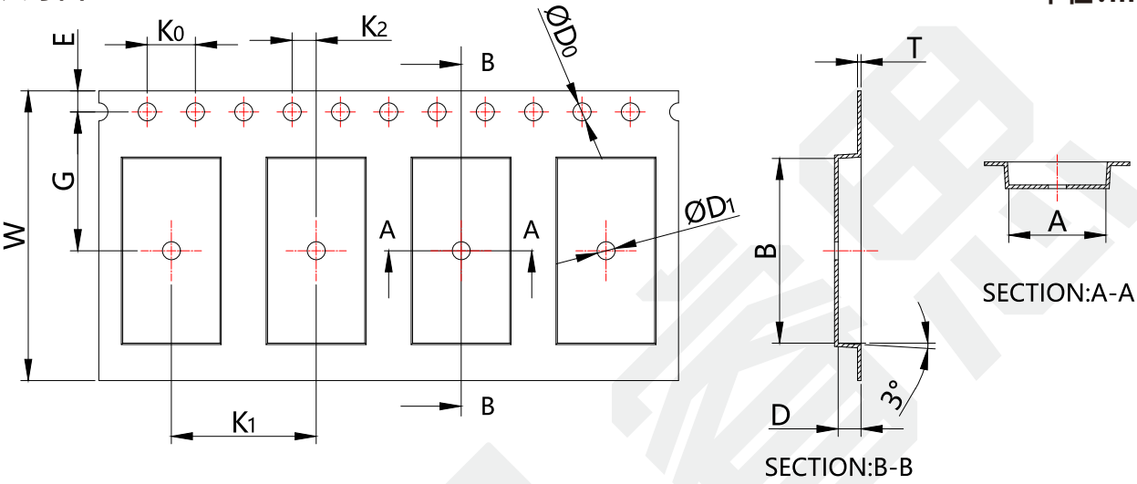
卷编带尺寸图
