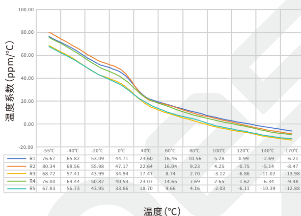
PEWM 系列 5930 规格 0.8mΩ 温度系数实测数据表
