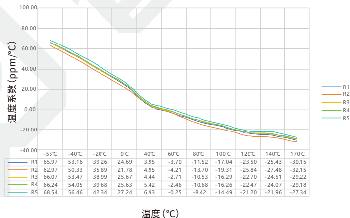
PEWM 系列 5930 规格 1.0mΩ 温度系数实测数据表
