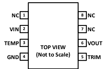
图 2. 8 引脚 SOIC
