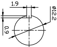
安装尺寸 (Mounting)
