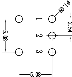
安装孔尺寸
