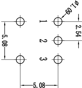
安装孔尺寸
