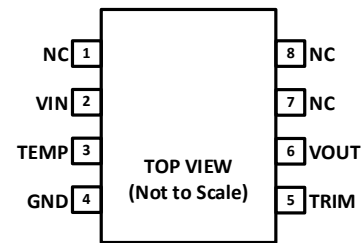
图 2. 8 引脚 SOIC
