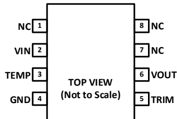
图 4. SOIC-8 引脚配置(顶视图)
