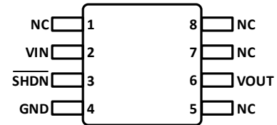
图 1. 8 引脚 MSOP
