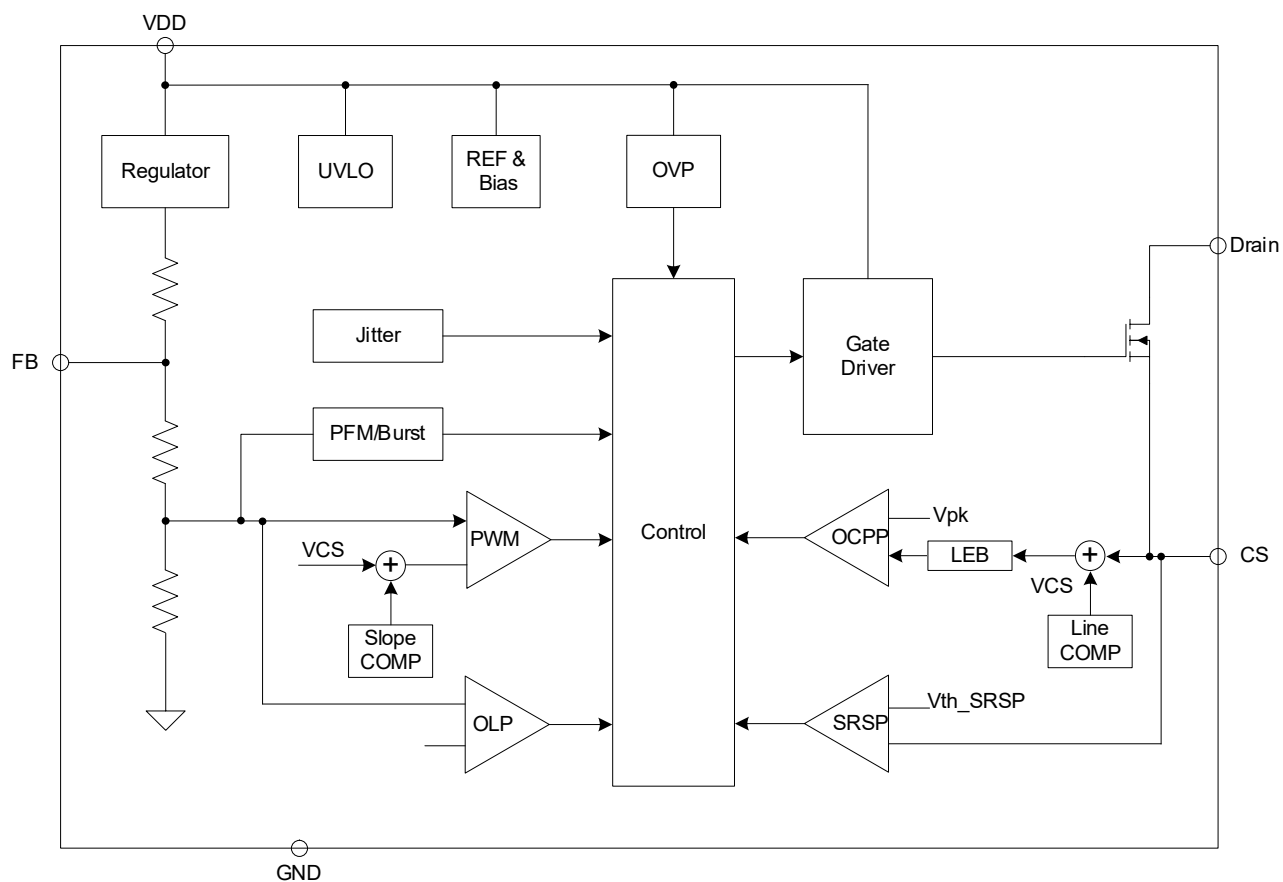
图 2 CM1764 功能模块框图
