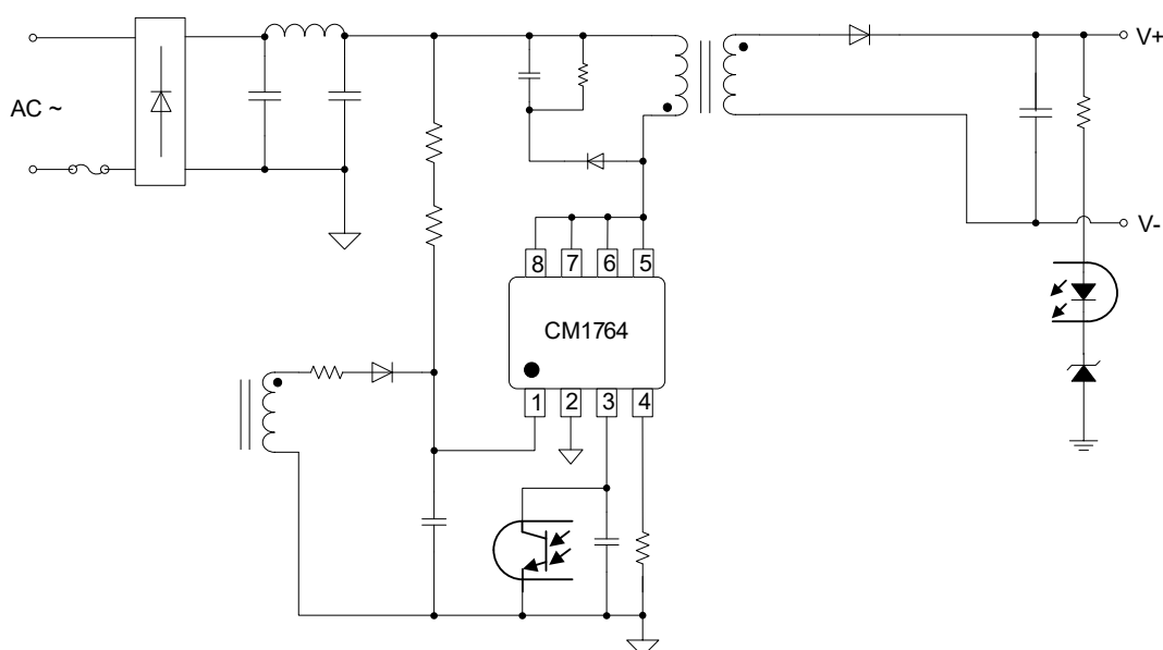
图 1 CM1764 典型应用电路
