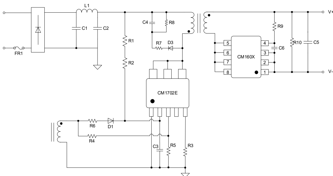
图 1 CM1702E 典型应用电路
