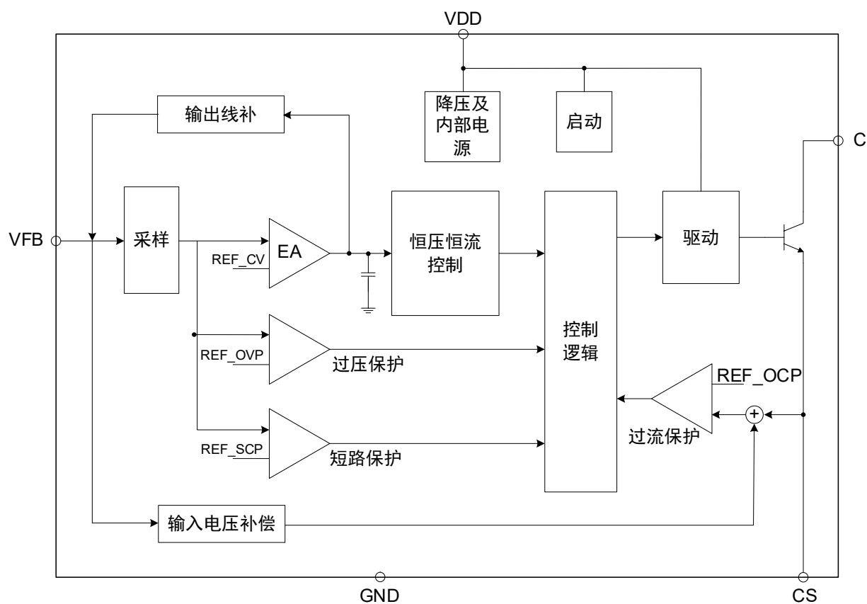
图 2 CM1702E 功能模块框图
