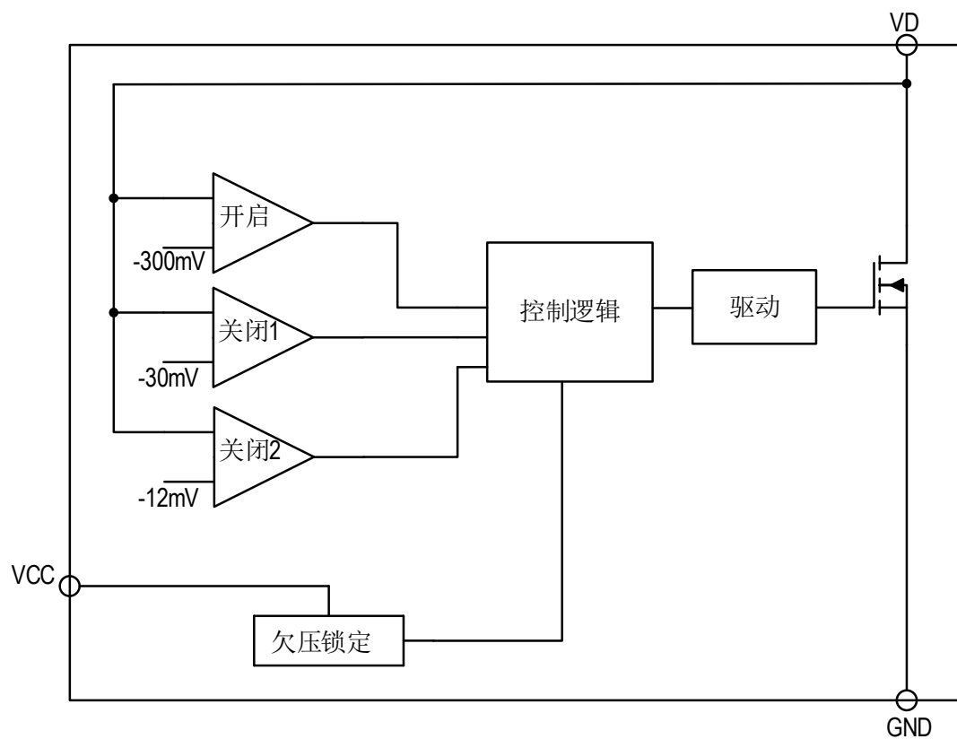
图 2 CM1600C 功能模块框图
