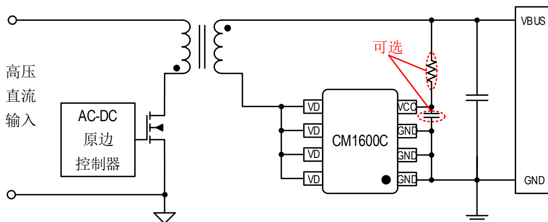
图 1 CM1600C 典型应用电路
