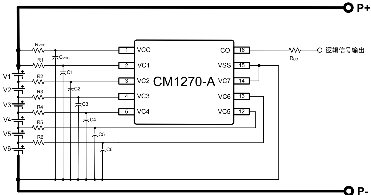
图 7 6 串应用原理图 2
