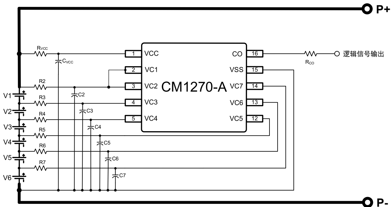
图 6 6 串应用原理图 1
