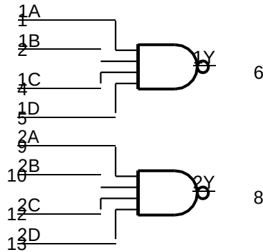
图 1 逻辑符号
