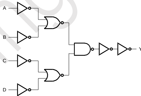
图 3 逻辑框图
