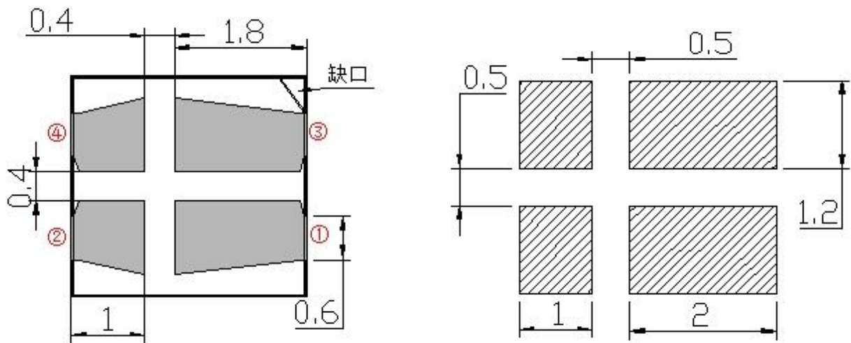
焊盘建议图
