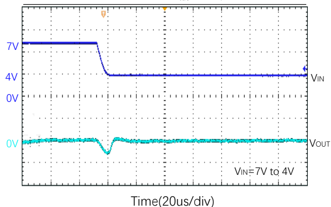
图10 输入跳变
