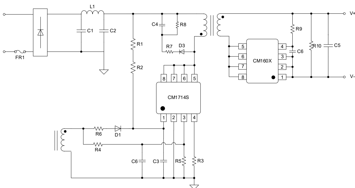
图 1 CM1714S 典型应用电路
