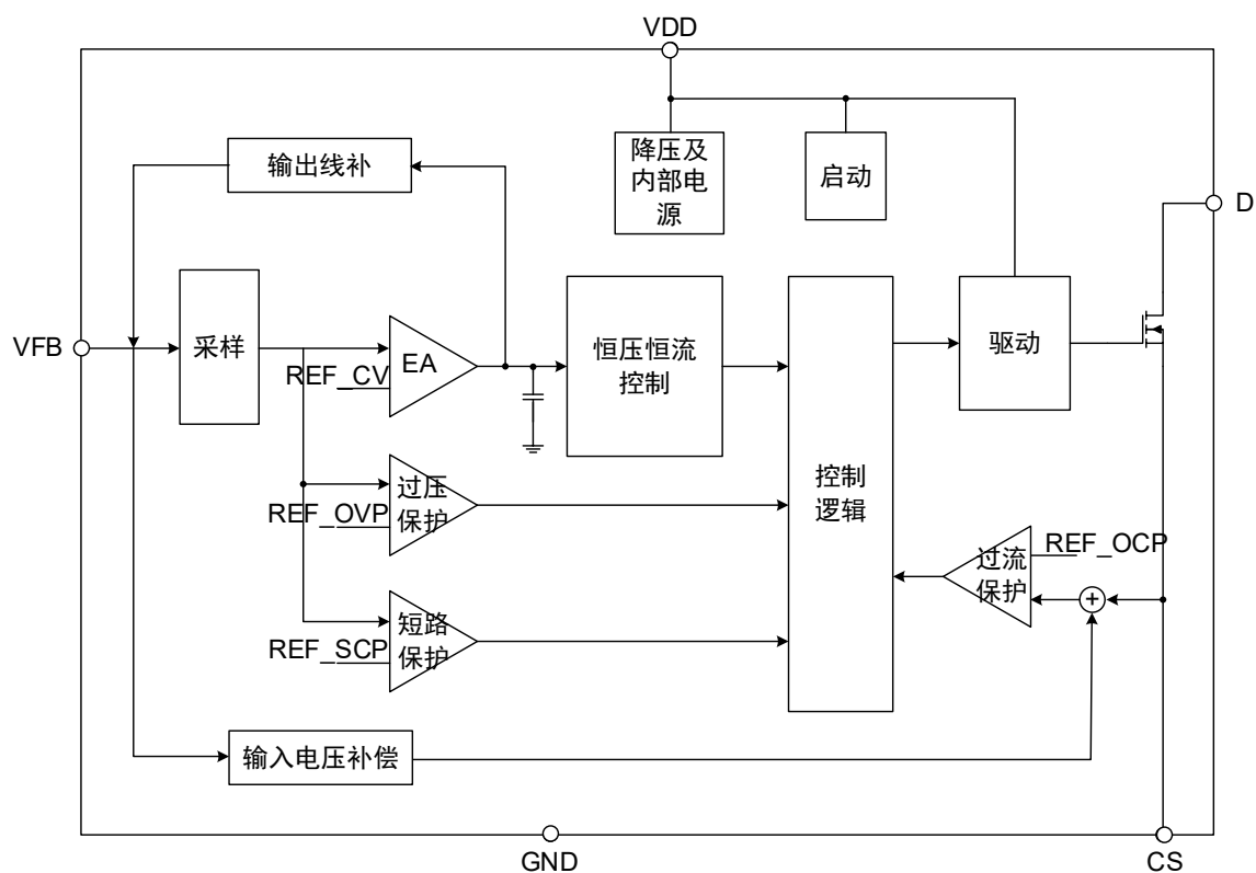
图 2 CM1714S 功能模块框图
