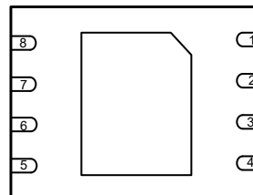
图 4 Bottom View
