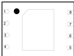
图 3 Top View
