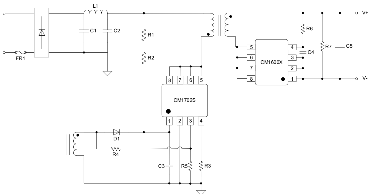
图 1 CM1702S 典型应用电路
