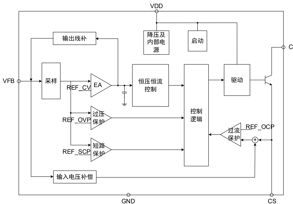
图 2 CM1702S 功能模块框图
