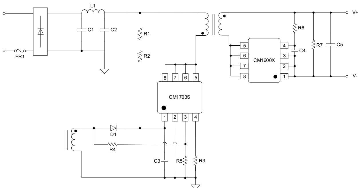
图 1 CM1703S 典型应用电路
