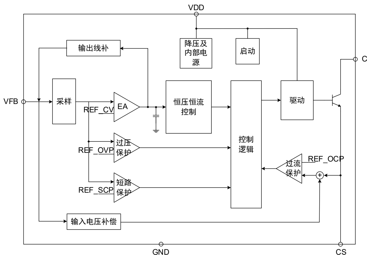
图 2 CM1703S 功能模块框图
