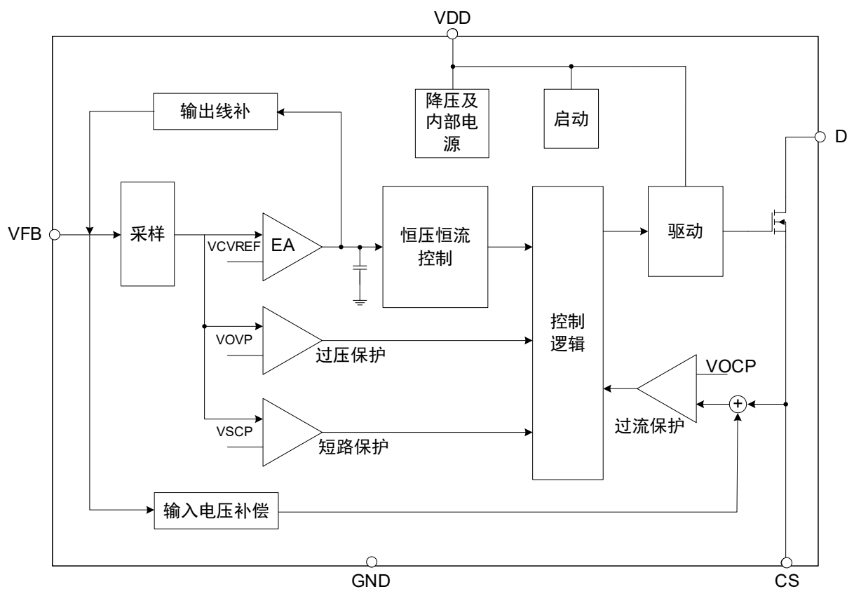
图 2 CM1714 功能模块框图
