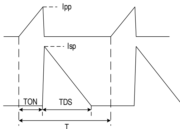
图 5 恒流工作原理图
