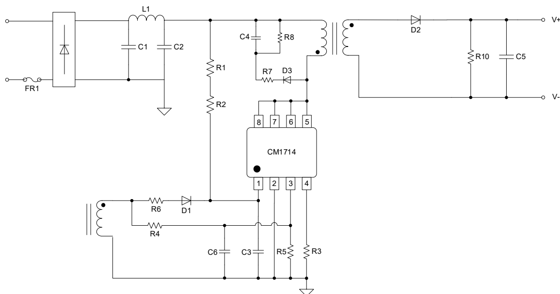
图 1 CM1714 典型应用电路
